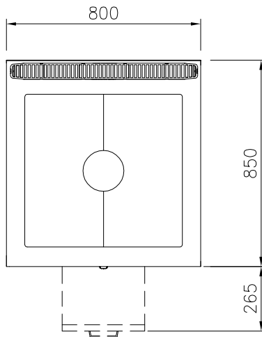
Boven aanzicht
